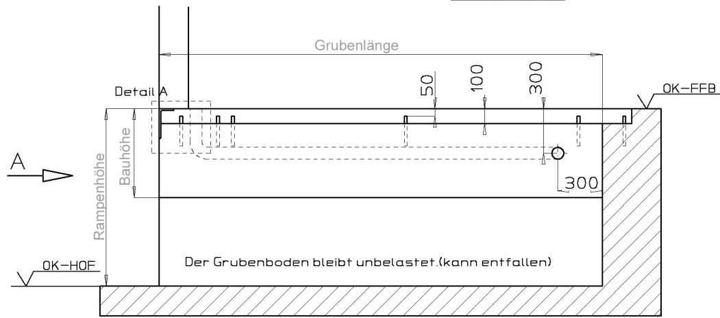
Schnitt B-B
